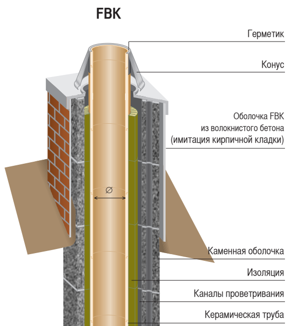
Оболочка FBK из волокнистого бетона с имитацией кирпичной кладки
