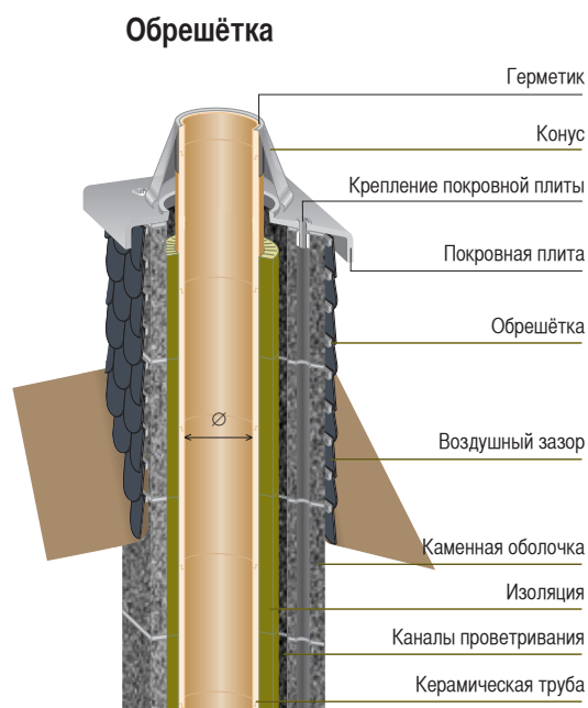
Выполняемая по месту обрешётка
