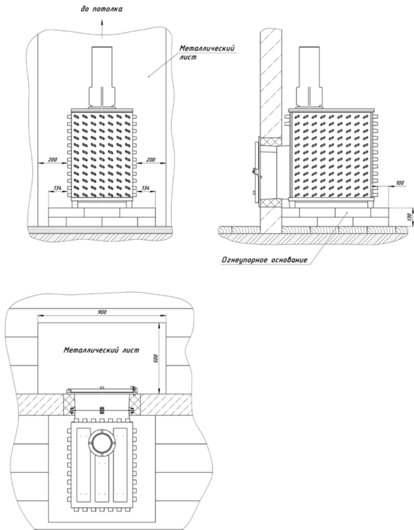
Рис.3 – Монтаж печи
